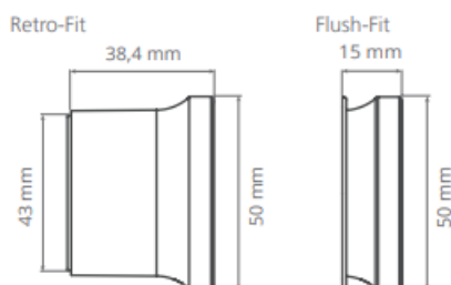
Seitenansicht
