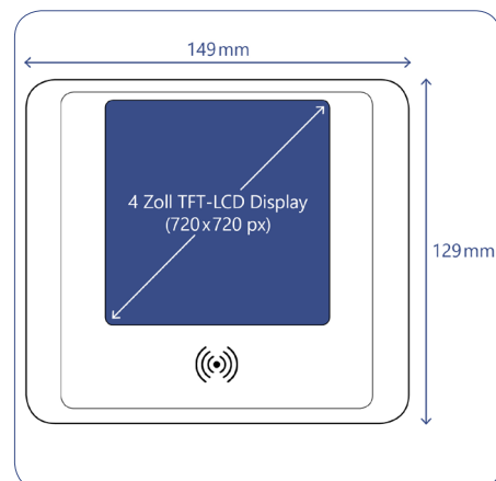
Abmessungen und Displaygröße des Terminals
